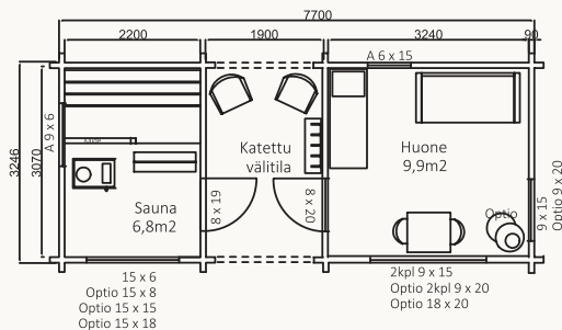
Saunamökki 25 A Välitila
