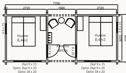
Vierasmaja 25 A Välitila
